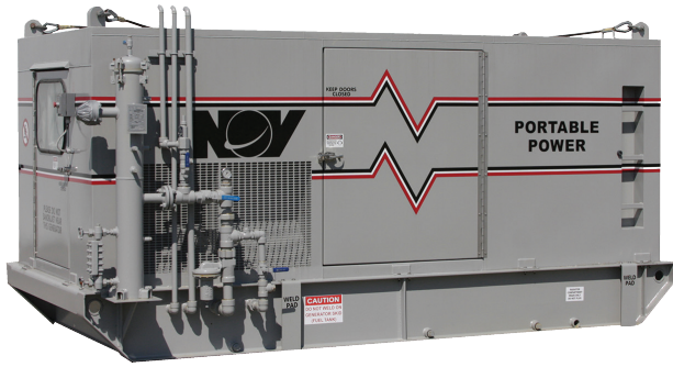
海上认证 防爆型 天然气发电机 & 海上认证 柴油发电机
