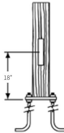
WBQ Elevation
